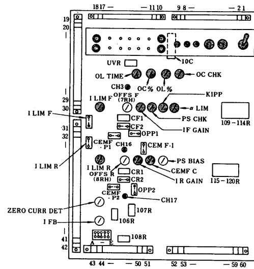
Fig. 12 Type JPDC-C021
