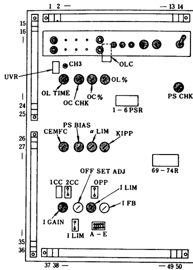
Fig. 11 Type JPDC-C020
