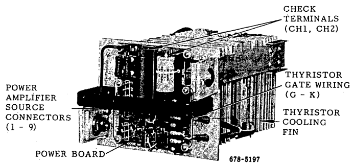
Fig. 10 Thyristor Module Type NPSB-X
